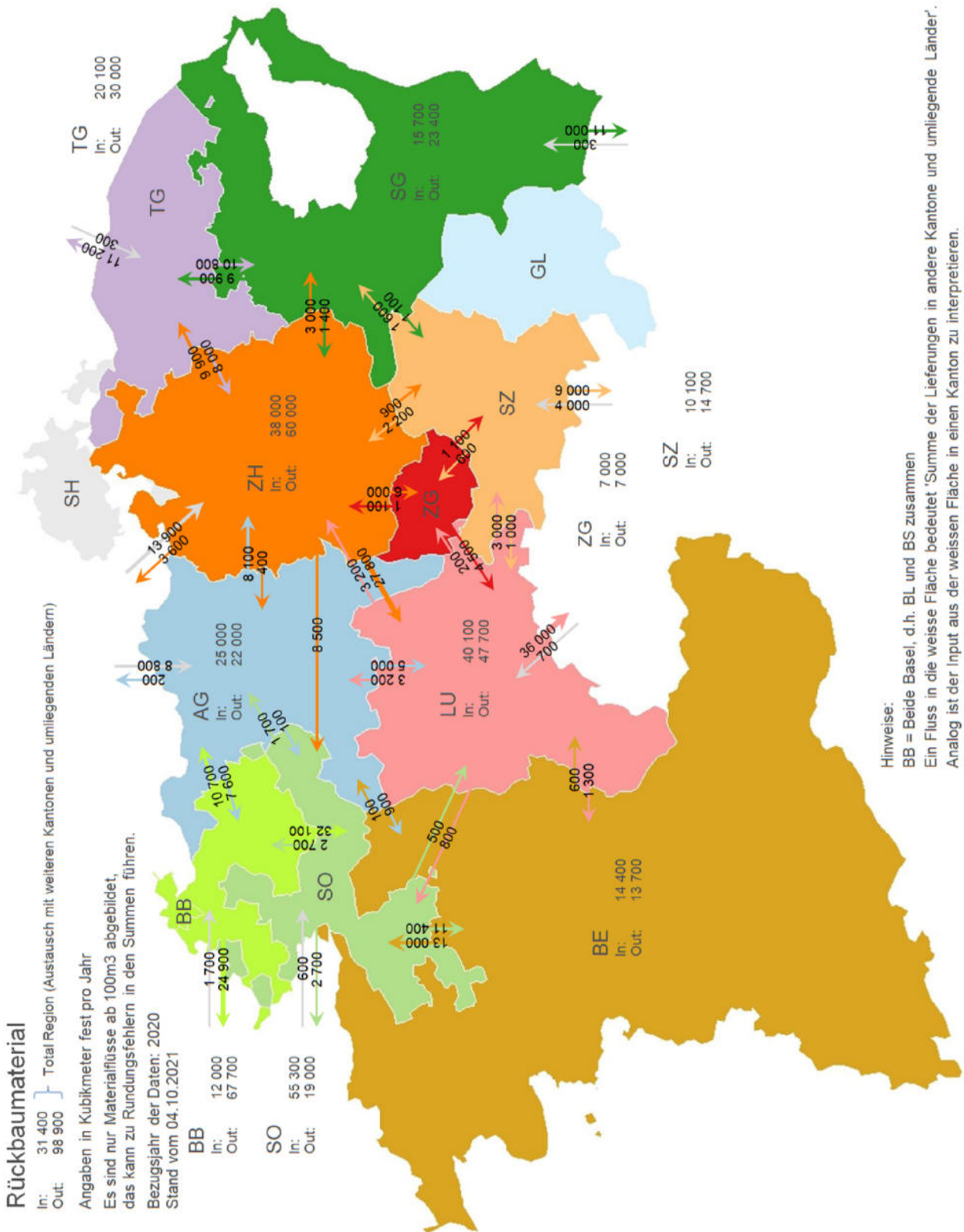
Abbildung 4: Rückbaumaterialflüsse über die Kantonsgrenzen im Jahr 2020. Die Werte unterhalb der Kantonsbezeichnungen bzw. unter dem Grafiktitel «Rückbaumaterial» entsprechen jeweils der Summe der Importe und Exporte.
