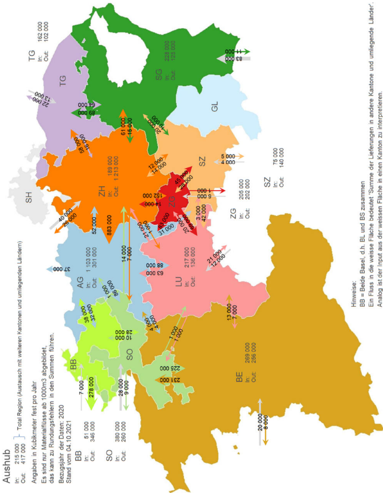
Abbildung 3: Aushubmaterialflüsse über die Kantonsgrenzen im Jahr 2020. Die Werte unterhalb der Kantonsbezeichnungen bzw. unter dem Grafiktitel «Aushub» entsprechen jeweils der Summe der Importe und Exporte.
