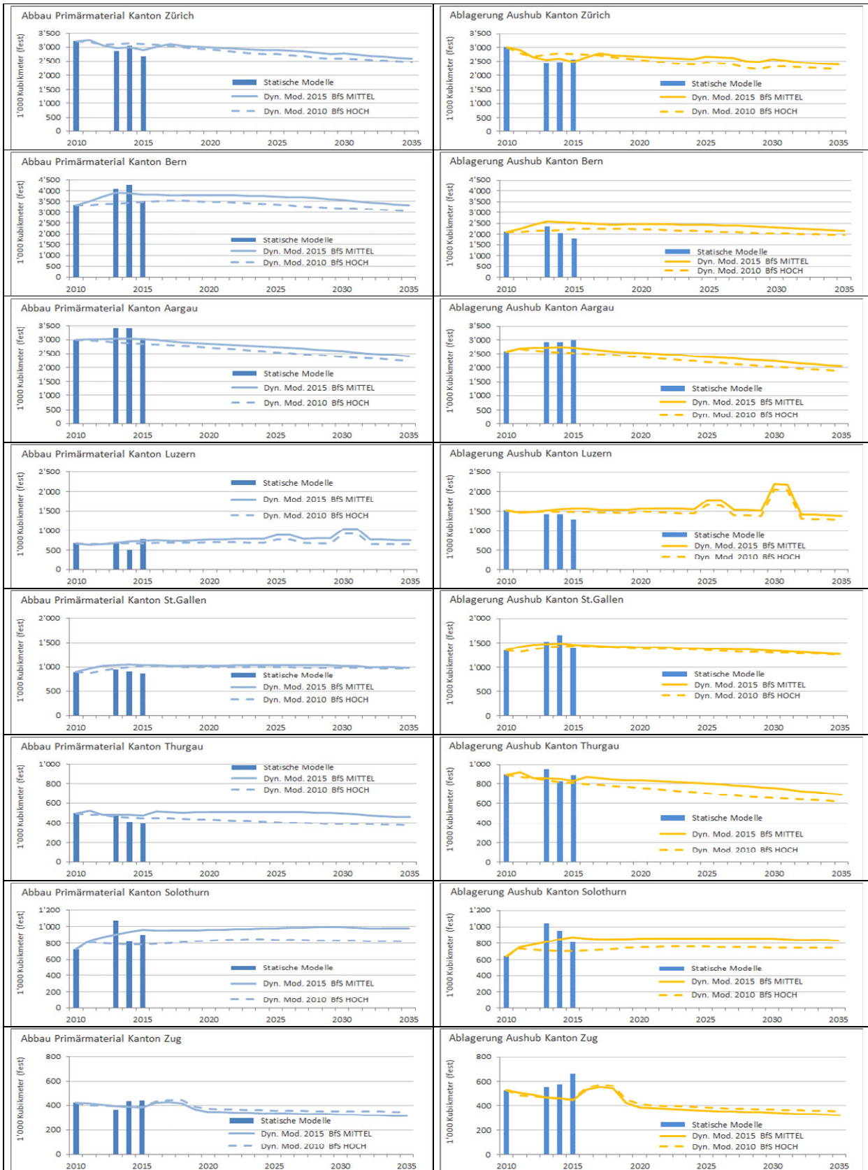
Abbildung 11: Entwicklung des Primärmaterialabbaus und der Aushubablagerung in den Kantonen ZH, BE, AG, LU, SG, TG, SO und ZG zwischen 2010 und 2035 (ausgezogene Linien: Szen. «Mittel, BFS 2015», gestrichelte Linien Szen. «Hoch, BFS 2010»), sowie die Daten aus den Modellierungen der Bezugsjahre 2010, 2013 - 2015. Angaben in 1000 m 3 fest.
