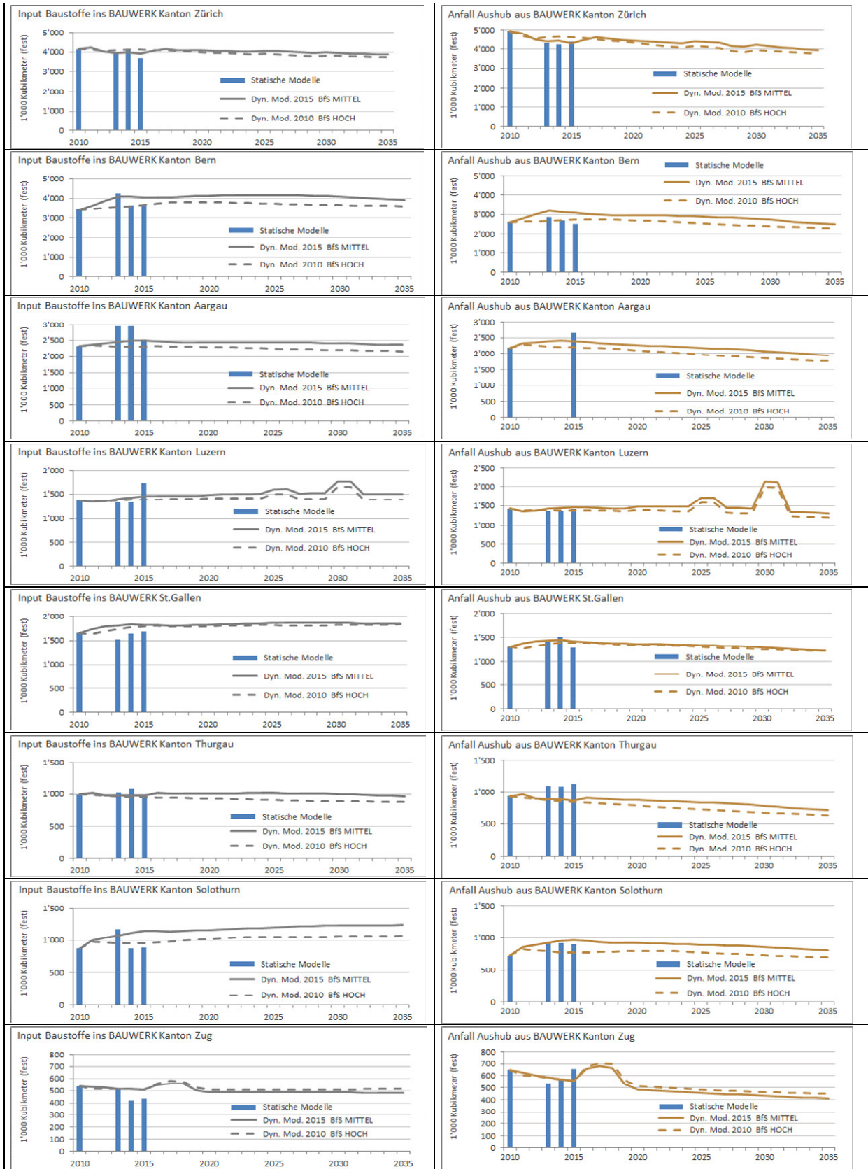
Abbildung 10: Entwicklung des Baustoffbedarfs und des Aushubanfalls in den Kantonen ZH, BE, AG, LU, SG, TG, SO und ZG zwischen 2010 und 2035 (ausgezogene Linien: Szen. «Mittel, BFS 2015», gestrichelte Linien Szen. «Hoch, BFS 2010»), sowie die Daten aus den Modellierungen der Bezugsjahre 2010, 2013 - 2015. Angaben in 1000 m 3 fest.
