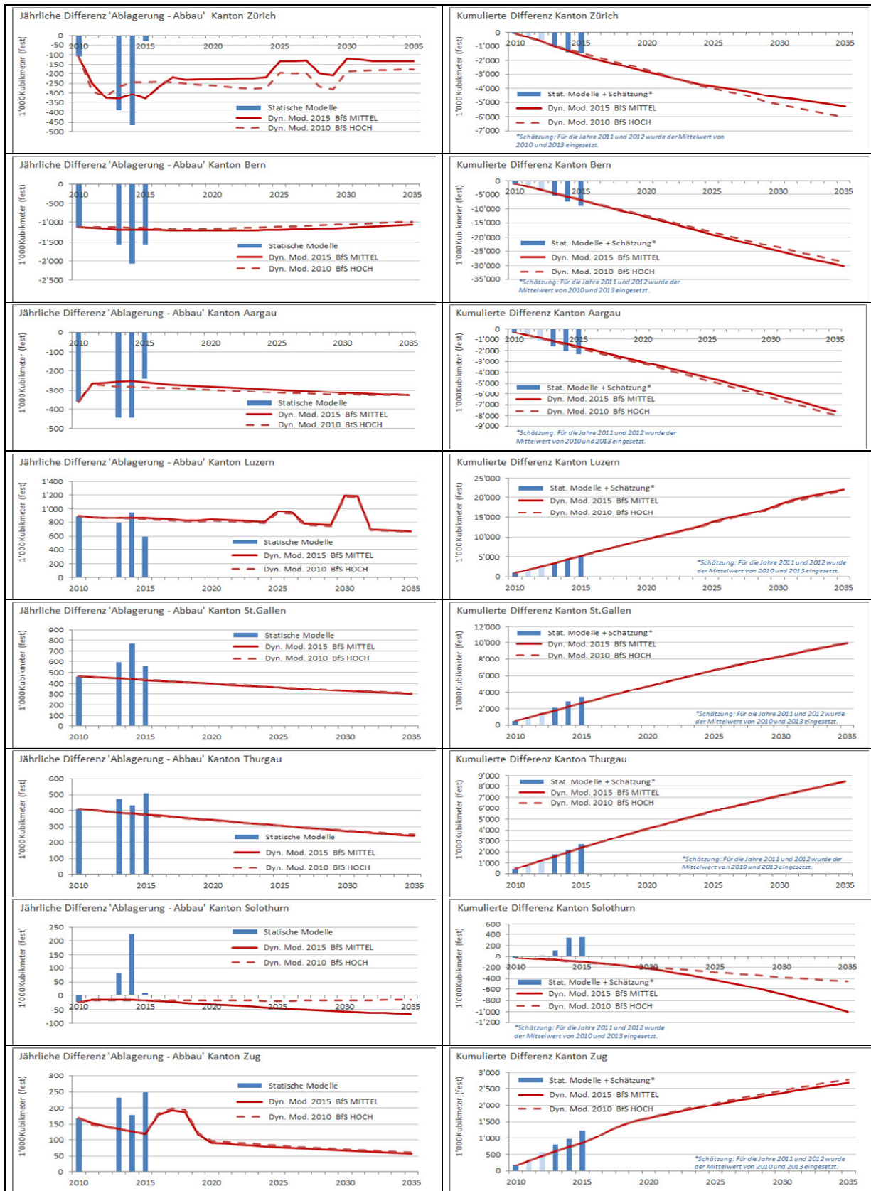
Abbildung 12: Entwicklung der jährlichen Differenz „Ablagerung – Abbau“ und die kumulierte Differenz in den Kantonen ZH, BE, AG, LU, SG, TG, SO und ZG zwischen 2010 und 2035 (ausgezogene Linien: Szen. «Mittel, BFS 2015», gestrichelte Linien Szen. «Hoch, BFS 2010»), sowie die Daten aus den Modellierungen der Bezugsjahre 2010, 2013 - 2015. Angaben in 1000 m3 fest.
