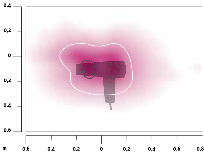
Magnetfeld eines Föhns. Unmittelbar an der Gehäuseoberfläche treten die stärksten Belastungen auf. Die Bedeutung der ausgezogenen Linien ist in der Farbskala unten dargestellt.
