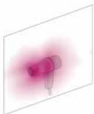
Magnetfeld eines Föhns. Unmittelbar an der Gehäuseoberfläche treten die stärksten Belastungen auf. Die Bedeutung der ausgezogenen Linien ist in der Farbskala unten dargestellt.
